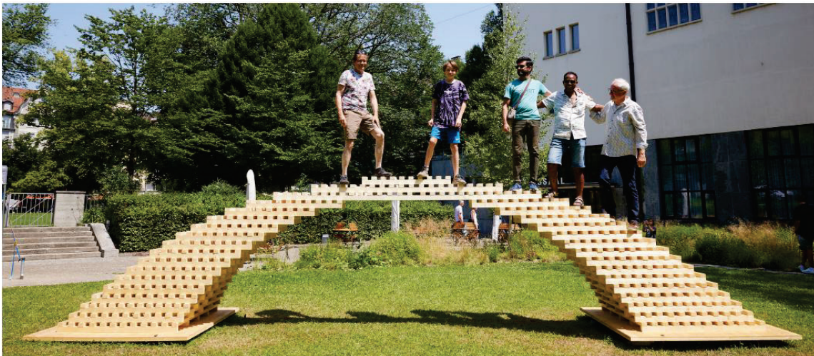
Brücke nach Fertigstellung bei einem Projekt in Luzern 2022
